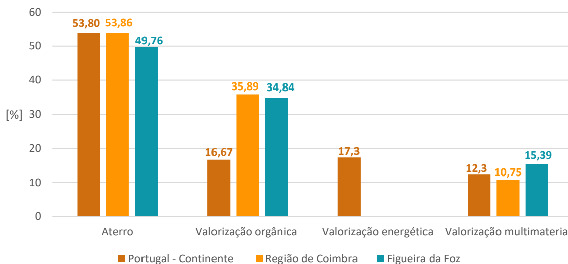
Figura 38. Resíduos urbanos geridos por tipo de destino no município da Figueira da Foz em comparação com a Região de Coimbra e Portugal-Continente (%), 2022.
