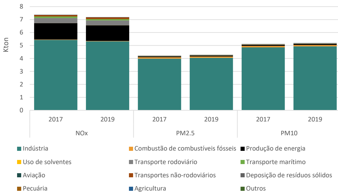
Figura 37. Emissão de gases para a atmosfera no município da Figueira da Foz, segundo o tipo de poluente e fonte de emissão (kton – quilotoneladas), 2017 e 2019.
