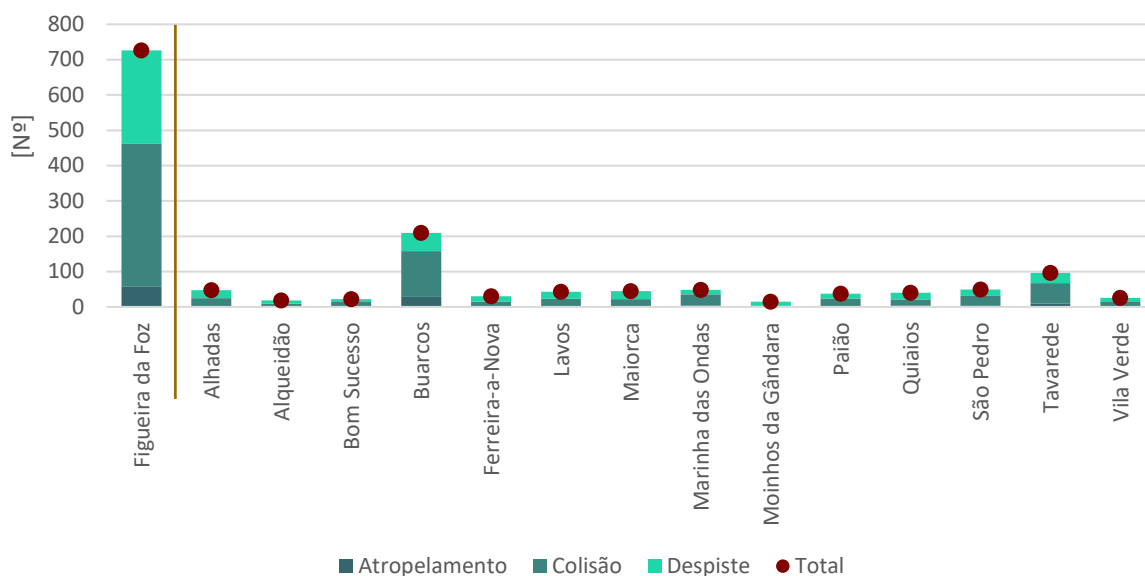
Figura 42. Acidentes de viação com vítimas no município da Figueira da Foz, segundo a natureza e freguesia (Nº), valores acumulados entre 2021 e 2023.
